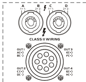
功率输出端
