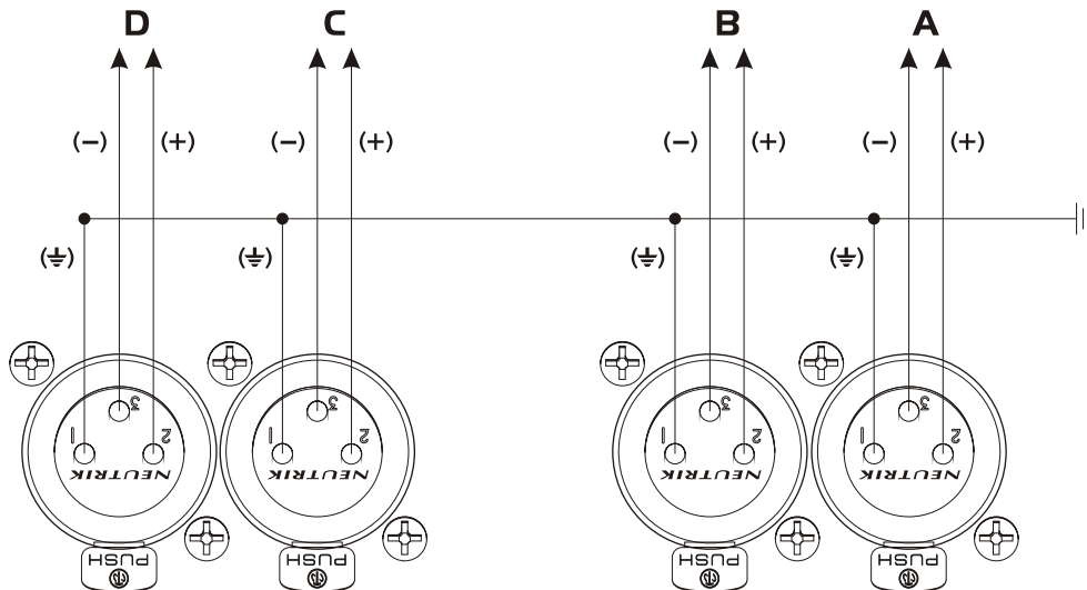
链接 LINK 平衡连接 母座 XLR
